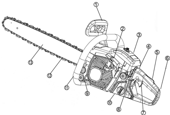
Fig. 6 – Componentes
