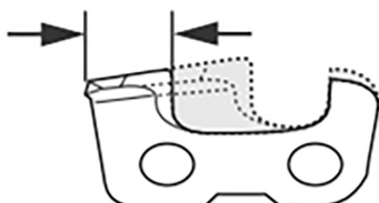
Fig. 39 - Diente con desgaste
