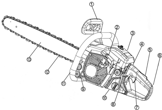
Fig. 6 – Componentes
