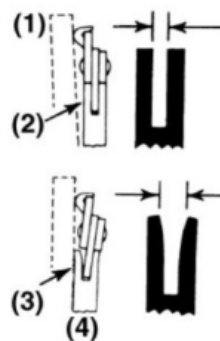
(1) Régua (2) Vão (3) Ausência de vão (4) Corrente torta
