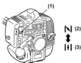
(1) Alavanca do afogador (2) Fechar (3) Abrir
