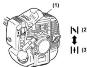
(1) Afogador (2) Fechado (3) Aberto
