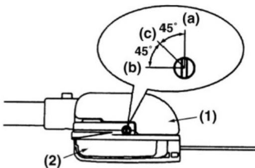
(1) Tanque de óleo (2) Capa da corrente
