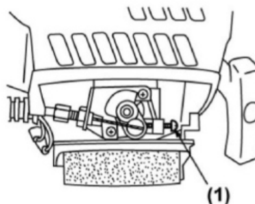
(1) Parafuso de ajuste de marcha lenta
