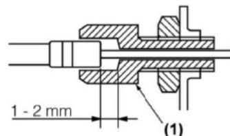
(1) Ajustador de cabo
